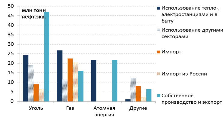
Рис. 6 Энергобаланс Украины
