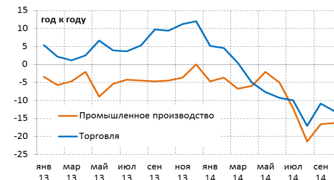
Рис. 1. Спад усиливается
